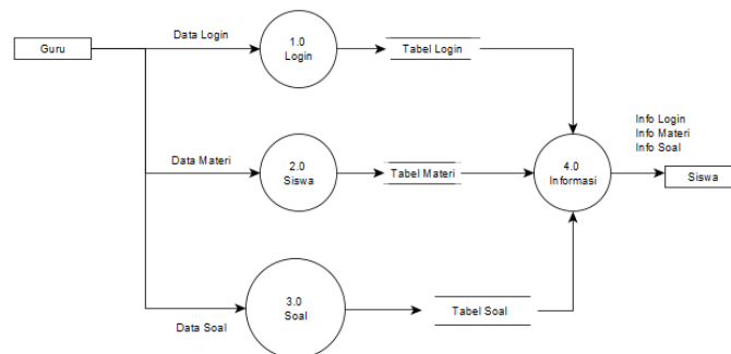
Gambar 2. DFD Level 1
